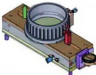
DOP GAUGE
